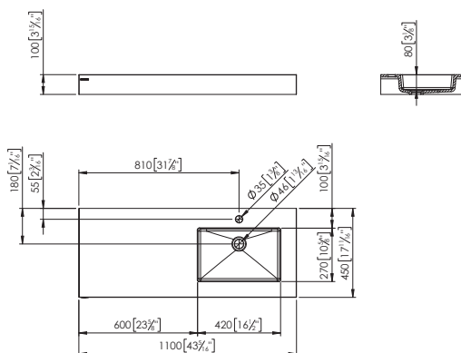
KOLE 110x45 (derecha · right · droite) (SIN REBOSADERO · WITHOUT OVERFLOW · SANS TROP-PLEIN)
