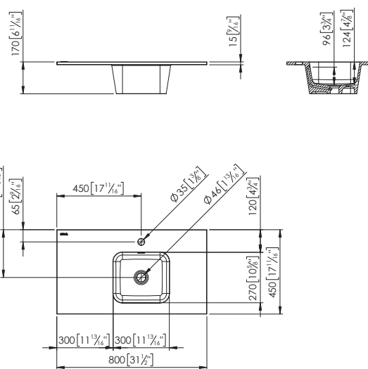
ENCIMERA MODUL DERECHA 120 MODUL 120 WORKTOP, RIGHT PLAN VASQUE MODUL DROITE 120
