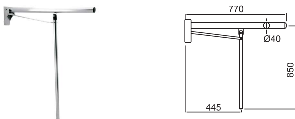
Vertical folding rail Barre rabattable verticale pour mur plâtre
