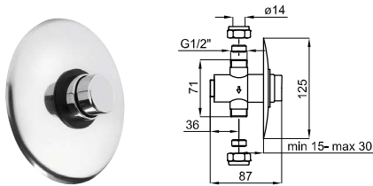
Concealed flush valve 1/2" for urinals. Fluxomètre poussoir encastré pour urinoir. Installation : encastré mur solide.
