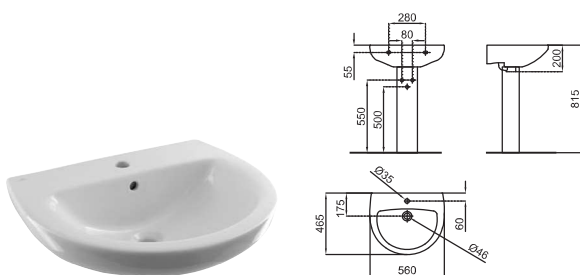
56 cm. wall hung basin with overflow and fixing kit 100041151 - N401150000. Lavabo 56 cm. avec trop plein. Avec fixations 100041151 - N401150000.
