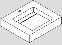
61 x 54 cm · 12h
