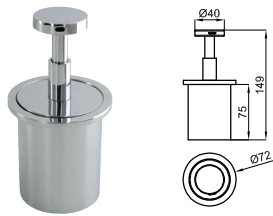
Concealed soap dispenser for countertop Diffuseur de savon sur plan
