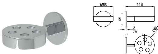
Wall mounted toothbrush holders Porte brosse à dent mural
