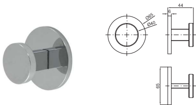
Robe hook Crochet
