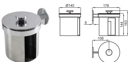
Roll holder with cover Porte-papier avec couvercle
