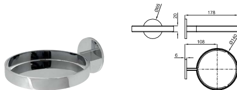
Soap dish for shower wall Porte-savon mural pour douche
