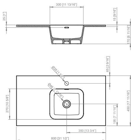
ENCIMERA MODUL DERECHA 80 MODUL 80 WORKTOP, RIGHT PLAN VASQUE MODUL DROITE 80
