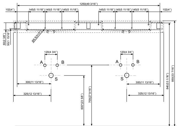
KOLE 70 (ESTANTE • SHELF • ÉTAGÈRE)
