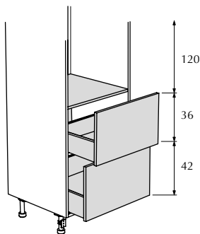
61 depth / profundidad / profondeur
