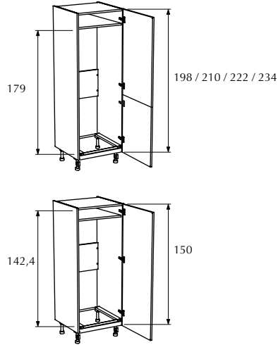
1 Carcass unit with hinges / Carcasa con bisagras / Caisson avec charnières.
