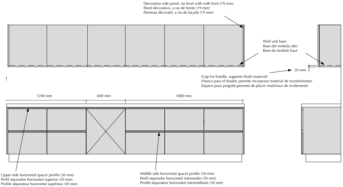
Front view Vista en alzado Vue du front
