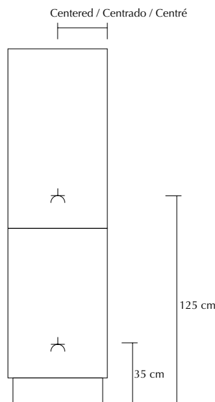
Tower unit for refrigerator and freezer Columna para frigorífico y congelador Colonne pour réfrigérateur et congélateur
