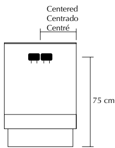
Base unit for oven and hob Bajo para horno y placa Bas pour four et plaque de cuisson
