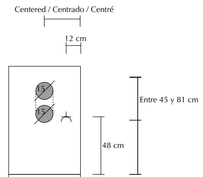
Installation set for dish washer Conexiones para lavavajillas Conexions pour lave-vaisselle
