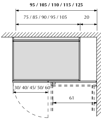
61 depth / profundidad / profondeur
