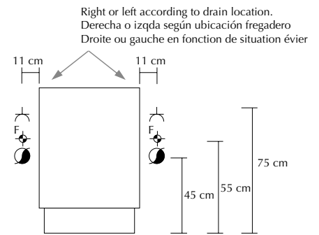
Installation set for dish washer Conexiones para lavavajillas Conexions pour lave-vaisselle
