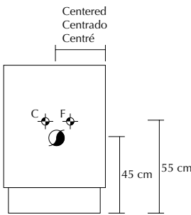
Base unit for sink Bajo para fregadero Bas pour évier
